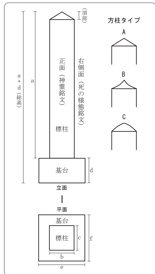
【図4】神霊碑形状図
